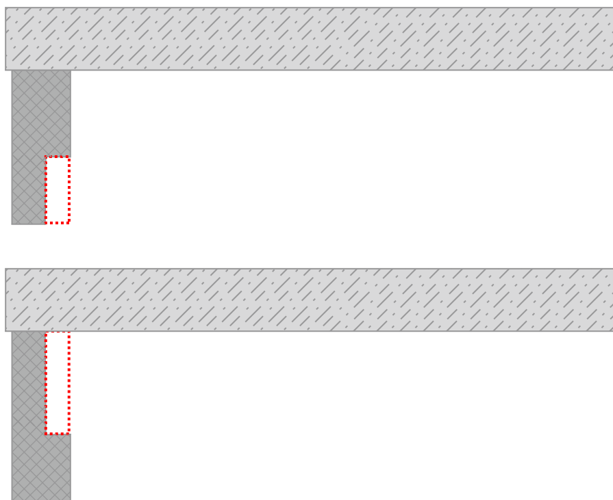
Рис. 10 Выравнивание притолоки
